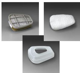
Kit 3M 60061: cartucho multigas 6006, retenedor 501 y filtro 5N11
