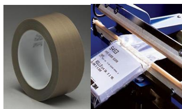
Cinta 3M de fibra de vidrio con teflón 5451
